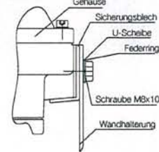
Montage Wandhalterung
