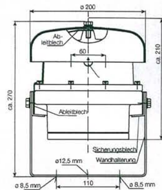
Montage Wandhalterung
