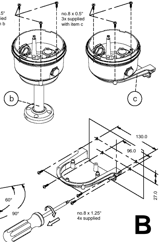
c) 90° Bracket M-400.000.01
