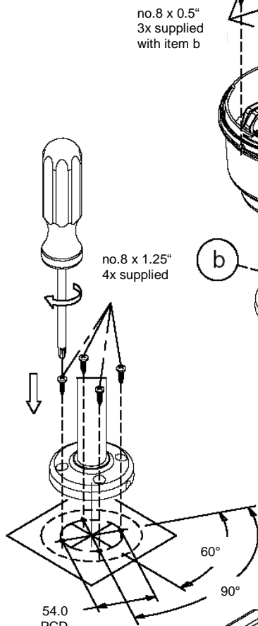
b) Pole Mount S-400.000.01
